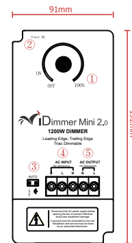
iDimmer mini 2.0
