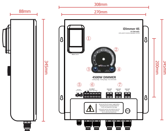
iDimmer 4S
